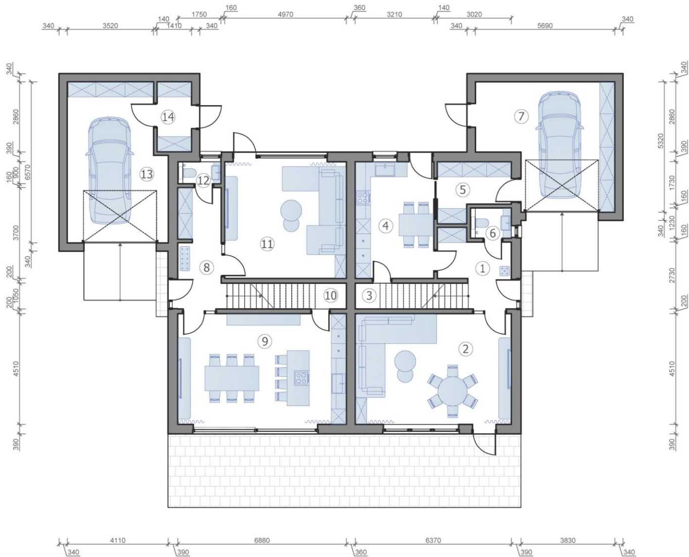
Grundriss 1. 1:100 (A-3)
